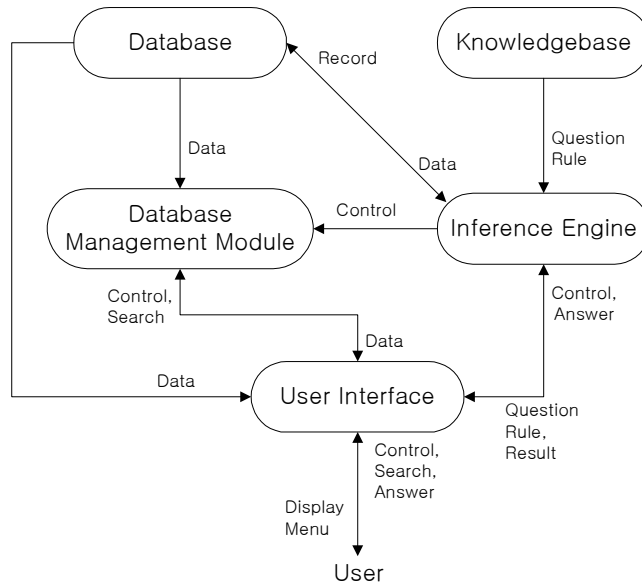
그림 2. SRAS 소프트웨어 구조
