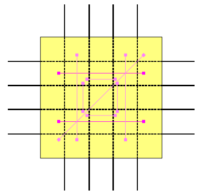
그림 5 LVDT 설치 위치
