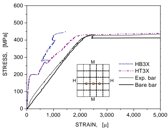
그림 20 원환방향 3번 철근으로부터 얻은 응력-변형률 곡선 (CP-B-S60-1)
