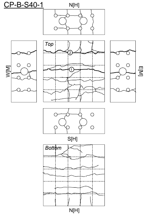
그림 7 실험체 CP-B-S40-1의 균열도
