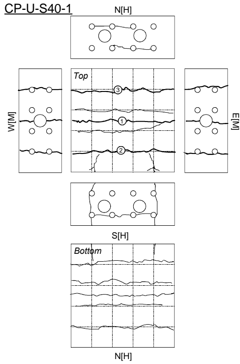
그림 6 실험체 CP-U-S40-1의 균열도
