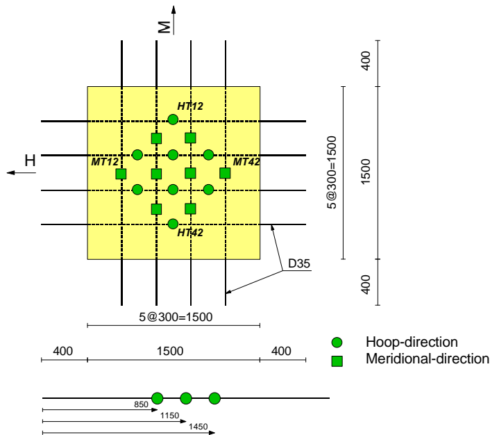
그림 4 변형률게이지 부착 위치
