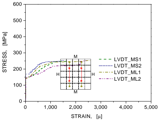
그림 18 자오선 방향 LVDT로부터 얻은 평균 응력-변형률 곡선 (CP-B-S60-1)
