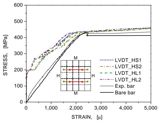
그림 17 원환방향 LVDT로부터 얻은 평균 응력-변형률 곡선 (CP-B-S60-1)
