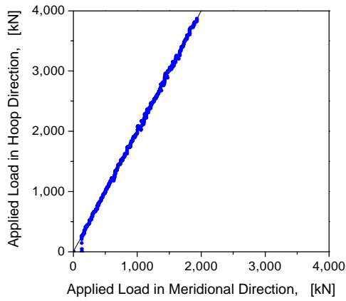
그림 16 원환방향 및 자오선 방향으로 도입된 하중 (H:M=2:1) (CP-B-S60-1)
