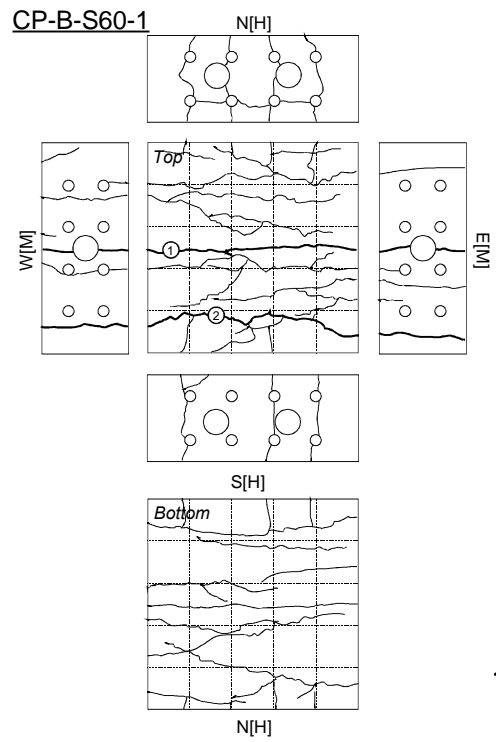
그림 9 실험체 CP-B-S60-1의 균열도
