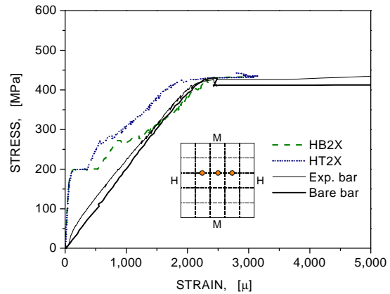
그림 19 원환방향 2번 철근으로부터 얻은 응력-변형률 곡선 (CP-B-S60-1)
