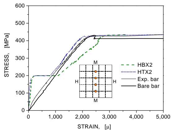
그림 21 원환방향 중앙위치 철근으로부터 얻은 응력-변형률 곡선 (CP-B-S60-1)
