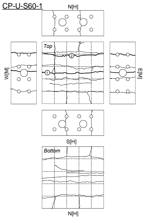
그림 8 실험체 CP-U-S60-1의 균열도
