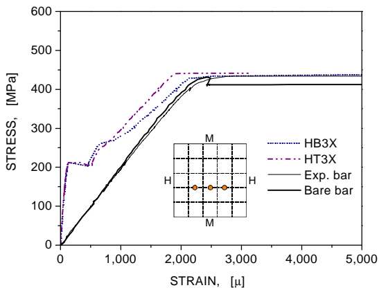
그림 14 원환방향 3번 철근으로부터 얻은 응력-변형률 곡선 (CP-B-S40-2)
