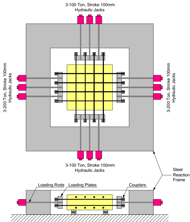
그림 3 가력시스템
