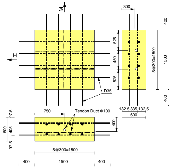
그림 2 실험체 제원
