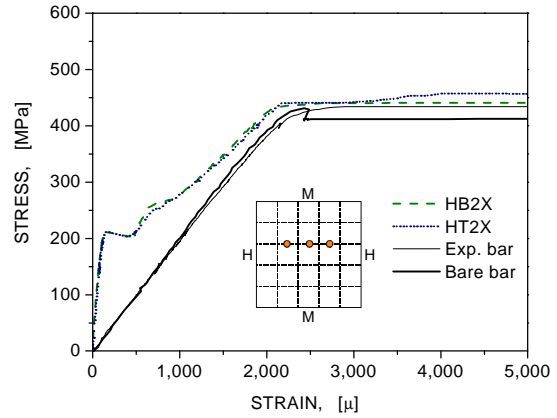
그림 13 원환방향 2번 철근으로부터 얻은 응력-변형률 곡선 (CP-B-S40-2)
