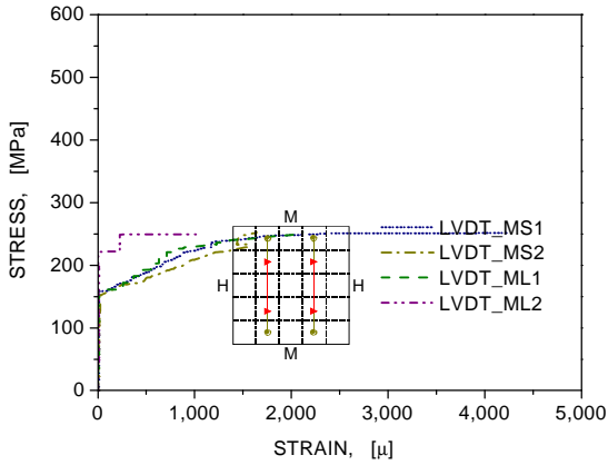
그림 12 자오선 방향 LVDT로부터 얻은 평균 응력-변형률 곡선 (CP-B-S40-2)
