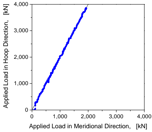
그림 10 원환방향 및 자오선 방향으로 도입된 하중 (H:M=2:1)
