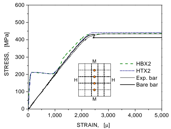
그림 15 원환방향 중앙위치 철근으로부터 얻은 응력-변형률 곡선 (CP-B-S40-2)
