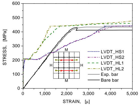
그림 11 원환방향 LVDT로부터 얻은 평균 응력-변형률 곡선 (CP-B-S40-2)
