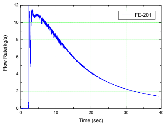
그림 5 Discharge Flow Rate Variation wrt Time 그림 6 Temperature Variations at R=40cm
