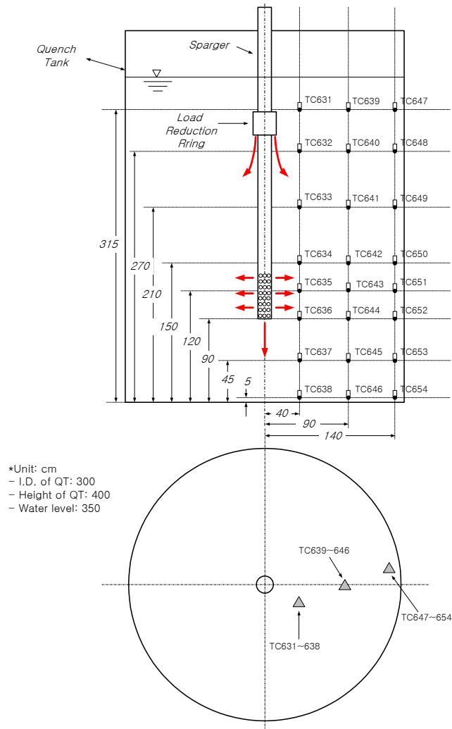
그림 2 Location of Thermocouples in the Quench Tank
