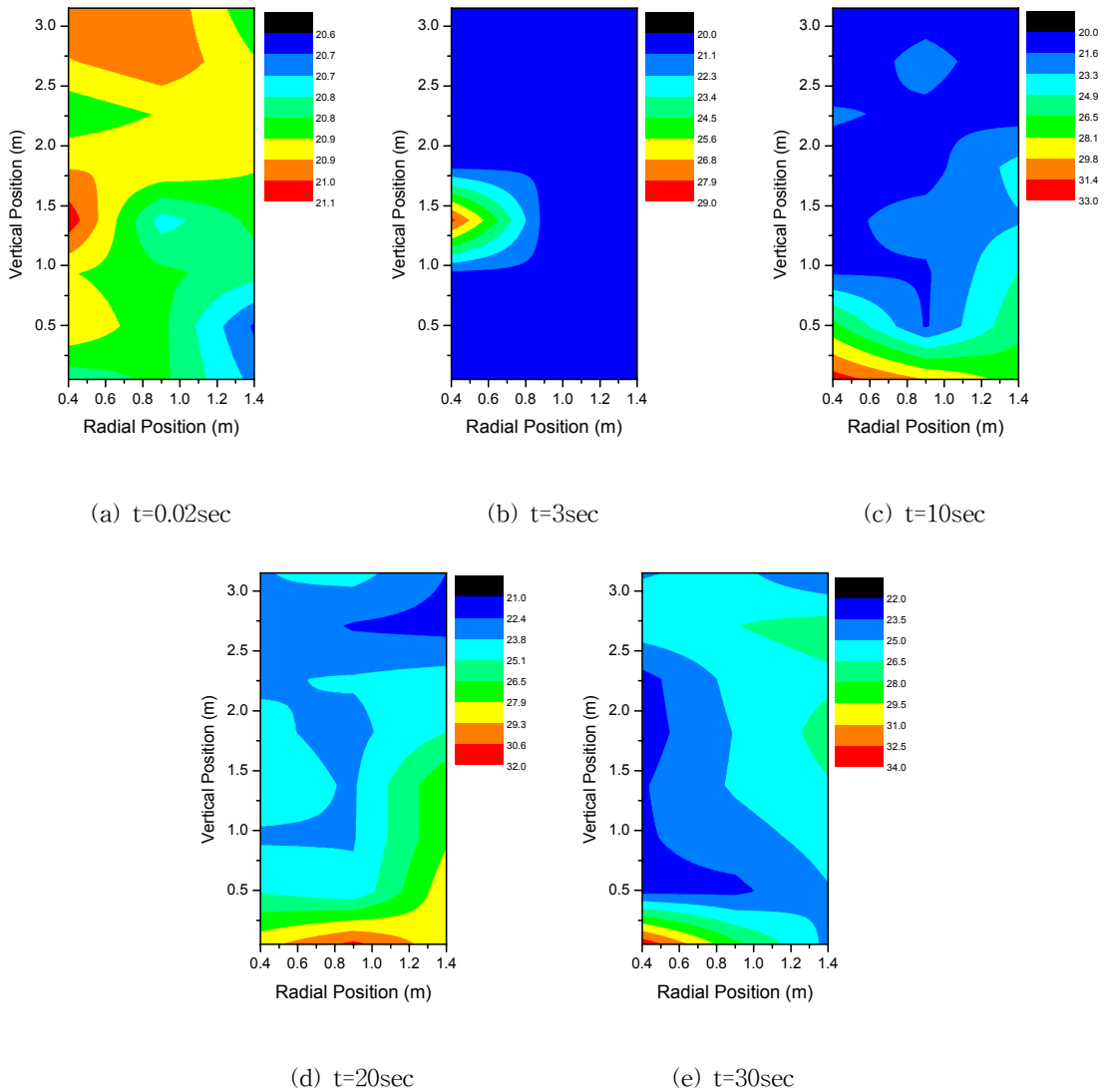
그림 9 Temperature Contour Variations
