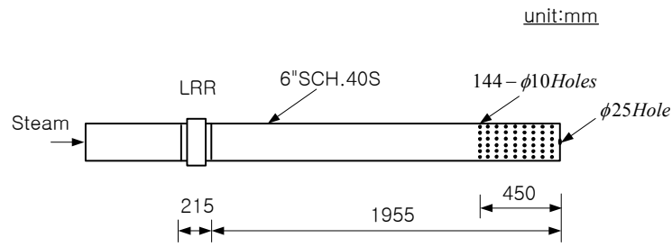
그림 3 Configuration of the APR1400 I-Sparger
