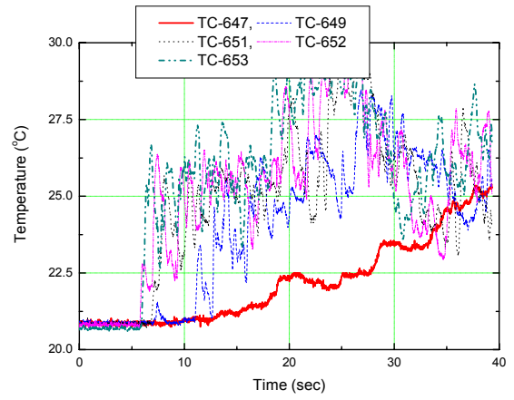
그림 8 Temperature Variations at R=140cm
