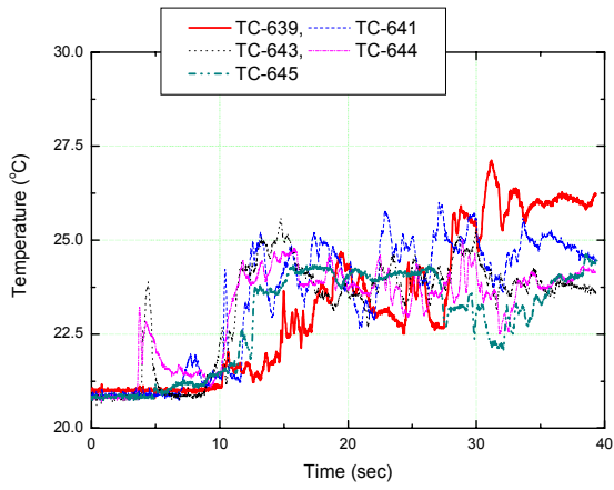
그림 7 Temperature Variations at R=90cm
